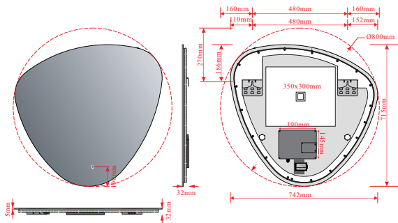
94.0022 DL-37-1-80 Ø800mm
