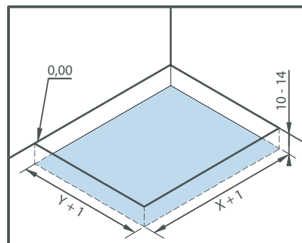
Montagevorbereitung Fertigfußboden mit Wannenfüße
